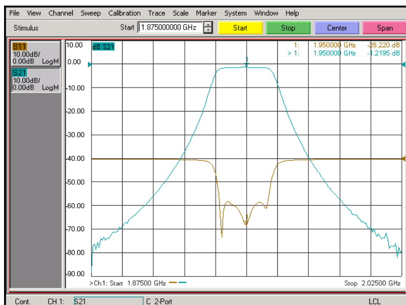
中心周波数付近でのフィルタ特性
